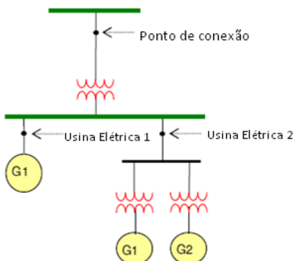
Figura 16 – Exemplo de compartilhamento de instalações entre geradores de energia Fonte: ONS (2011) 60
