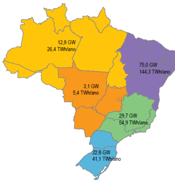
Figura 9: Potencial brasileiro de recursos eólicos 43 .
