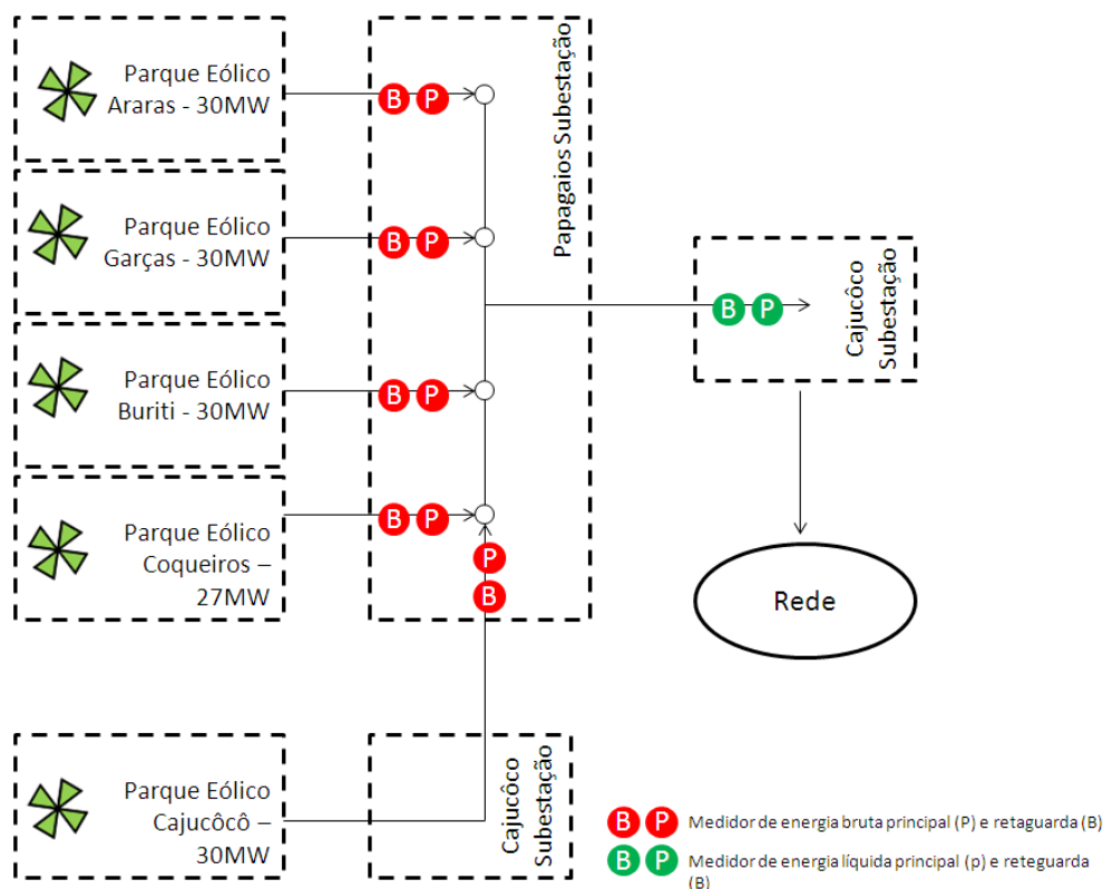
Figura 15 - Diagrama detalhando os pontos de medição do projeto.
