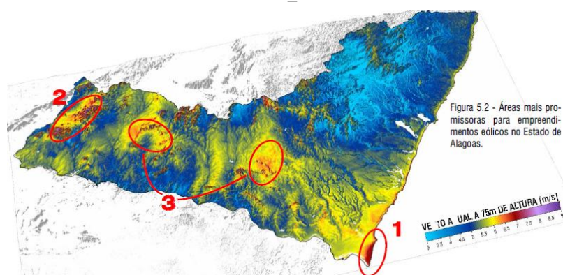
Figura 12- Potencial eólico de Alagoas. Fonte: Eletrobras – Atlas do Potencial Eólico de Alagoas.
