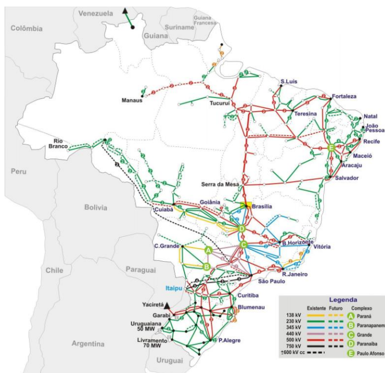
Figura 14 – Sistema Interligado Nacional. (Fonte: Operador Nacional do Sistema Elétrico)
