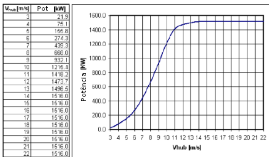
Figura 6 – Potência gerada como função da velocidade do vento.
