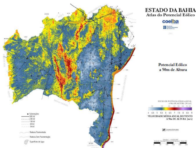
Figura 11 – Potencial eólico do estado da Bahia. Fonte: COELBA - Atlas do Potencial Eólico do estado da Bahia.
