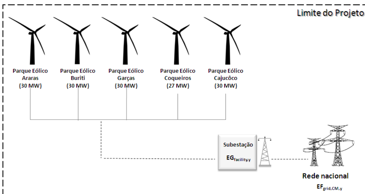
Figura 7 – Fluxograma simplificado do limite do projeto
