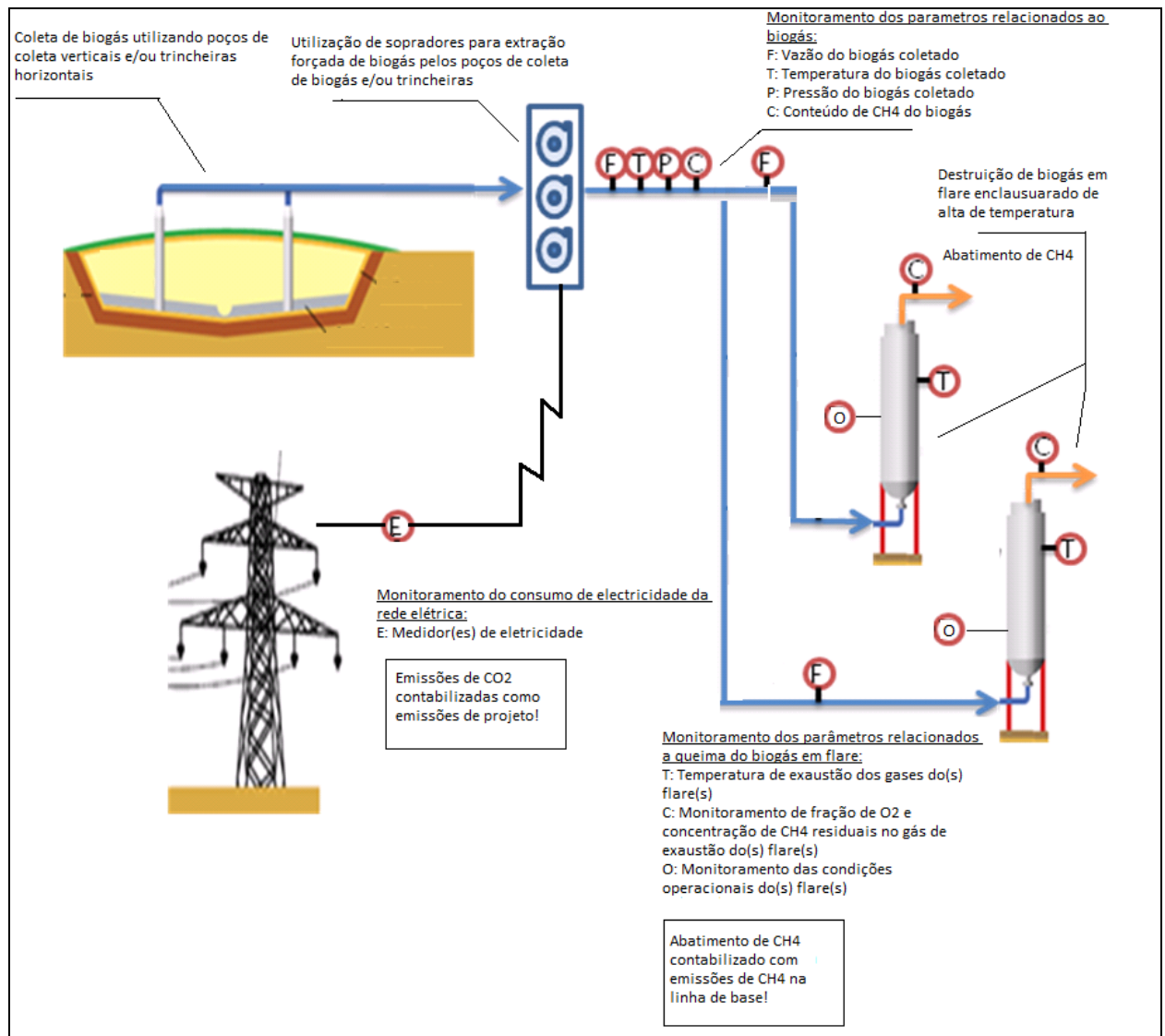
Fluxograma esquemático: delimitação do limite do projeto para a atividade de projeto
