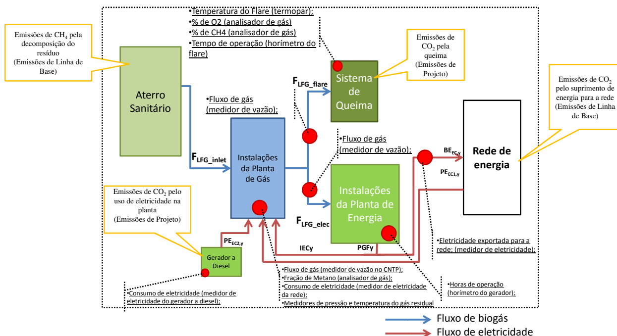
Figura 12 – Fluxograma do limite do projeto
