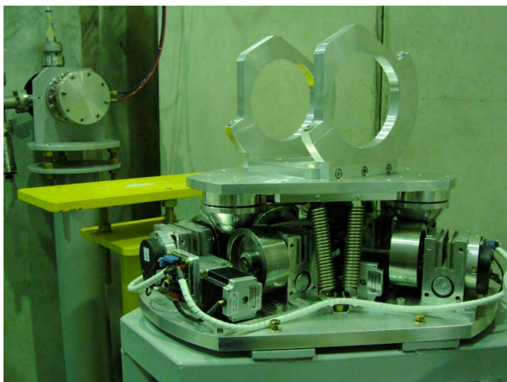
Figura 2: Sistema hexápode
