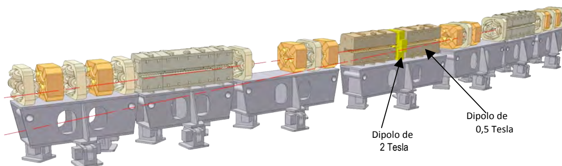
Figura 4: Magnetos de um arco acromático de SIRIUS
