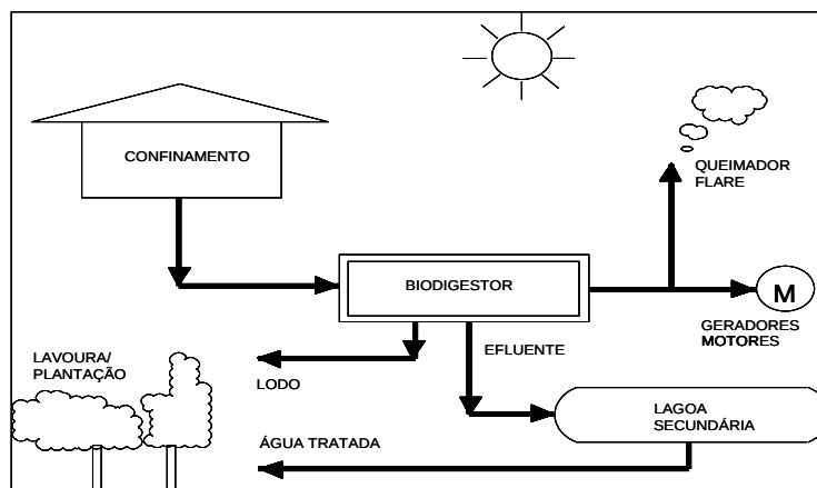
Figura A2. Esquema do Sistema de Tratamento
