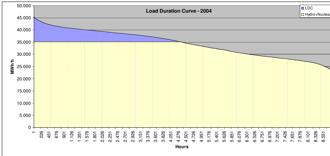
LOAD CURVE ING SSEMW, 2004
