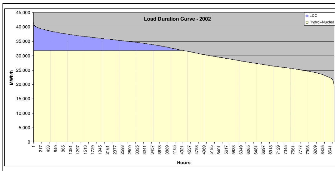
LOAD CURVE ING SSEMW, 2002
