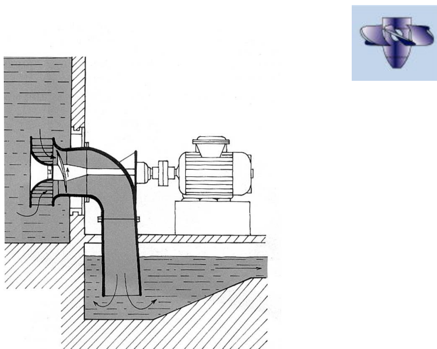
Figura 2 – Turbina Kaplan (Fontes: Alstom, http://www.alstom.com.br/ )
