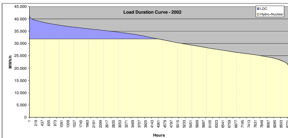
Figura 9 - Curva de duração da carga para o sistema S-SE-CO, 2002
