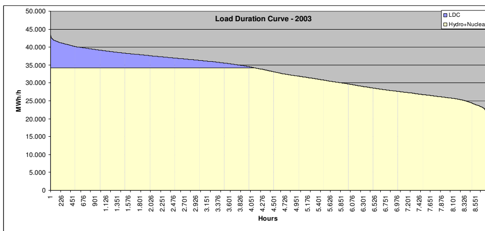
Figura 10 - Curva de duração da carga para o sistema S-SE-CO, 2003
