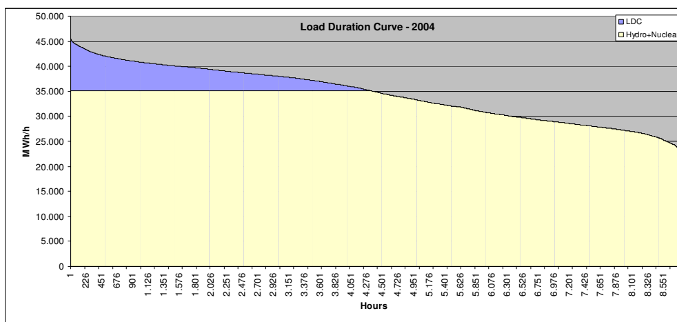
Figure 11 – Curva de duração da carga para o sistema S-SE-CO, 2004
