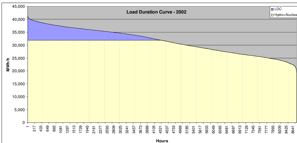
Curva de duração de Carga para o sistema S/SE/CO, 2002
