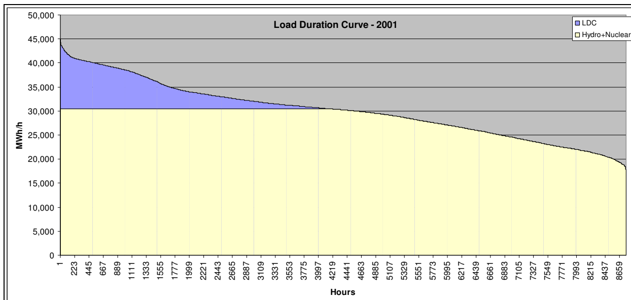
Curva de duração de Carga para o sistema S/SE/CO, 2001
