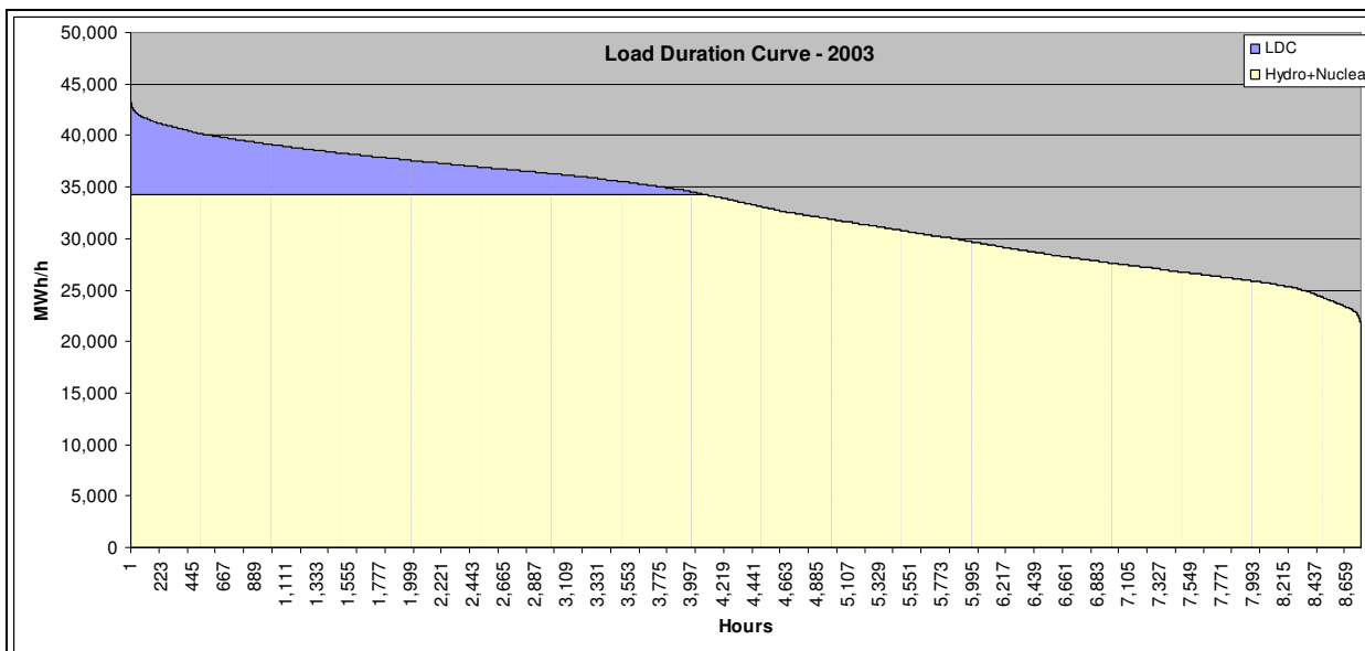
Curva de duração de Carga para o sistema S/SE/CO, 2003
